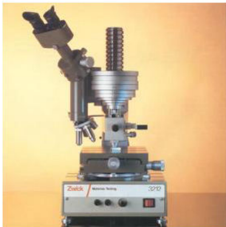
Slika 25. Tvrdomijer Zwick
