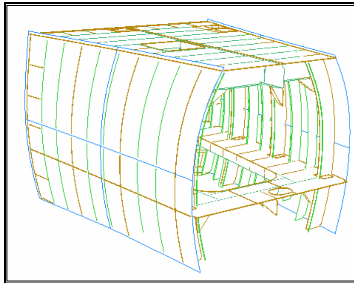
Slika 46. Pramčana sekcija 4012
