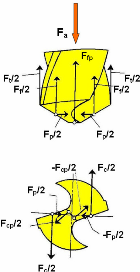
Slika 23. Sile rezanja kod bušenja [9]
