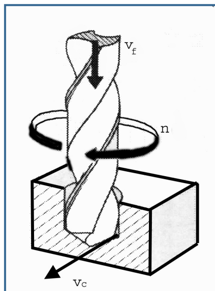
Slika 15 . Shematski prikaz bušenja spiralnim svrdlom [6]
