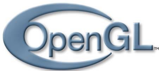
Slika 12 Logotip OpenGL-a
