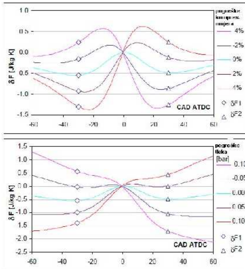
Slika 8. Promjena funkcije gubitaka \delta F uz prisutnost pogreške kompreijskog omjera (gore) i pogreške tlaka (dolje) (ciklus tlaka postupno prema LPP=0 , \delta\vartheta = 1^\circ KV )
