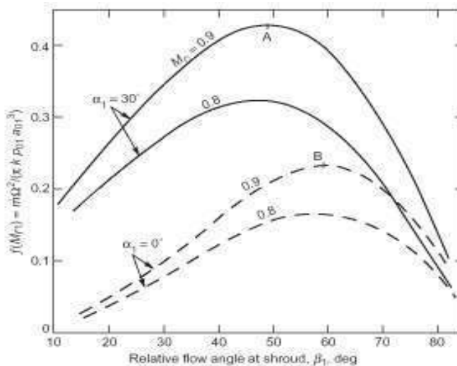
Slika 2.5 a) prikazuje varijaciju funkcije masenog protoka centrifugalnog kompresora sa i bez usmjeravajućih lopatica.
