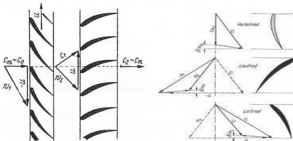
Tokovi brzina stupnja aksijalnog kompresora 2.8 b)
