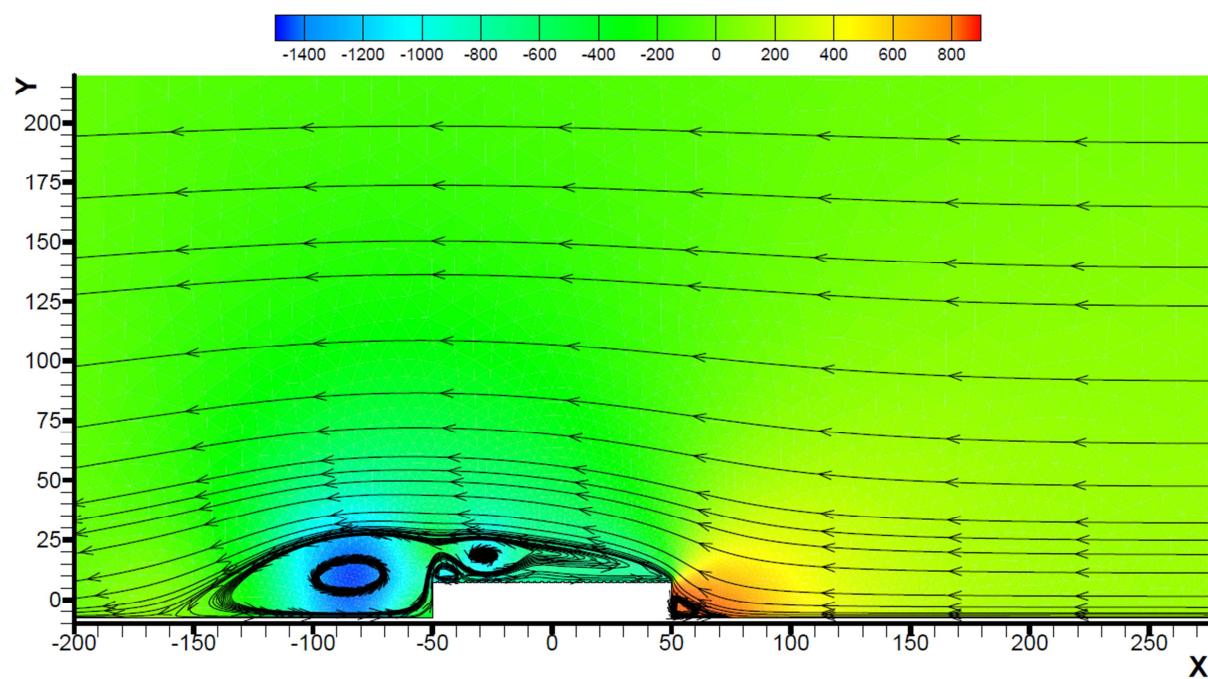
Slika 110. Strujnice simulacije I sa suprotnim smjerom strujanja
