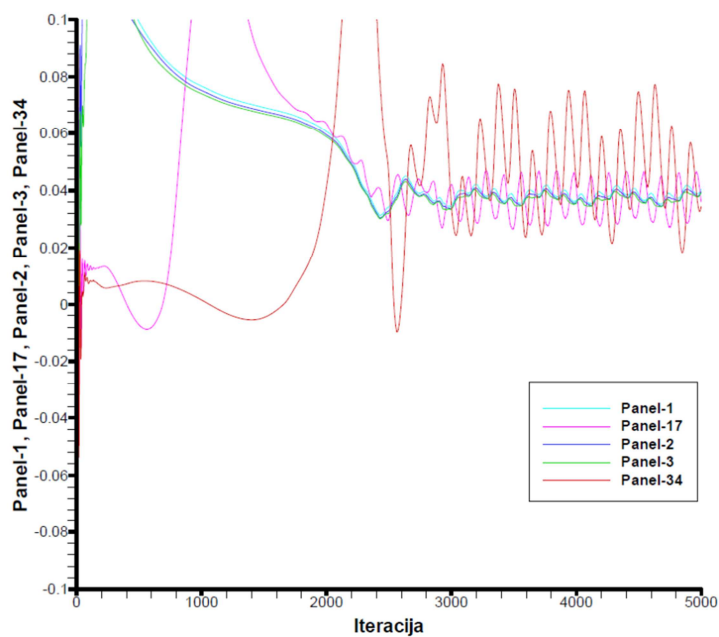
Slika 43. Konvergencija koeficijenta C_L za 1., 17., 32., 33. i 34. reda panel u simulaciji D
