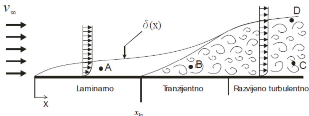
Slika 12. Granični sloj uz ravnu ploču [14]
