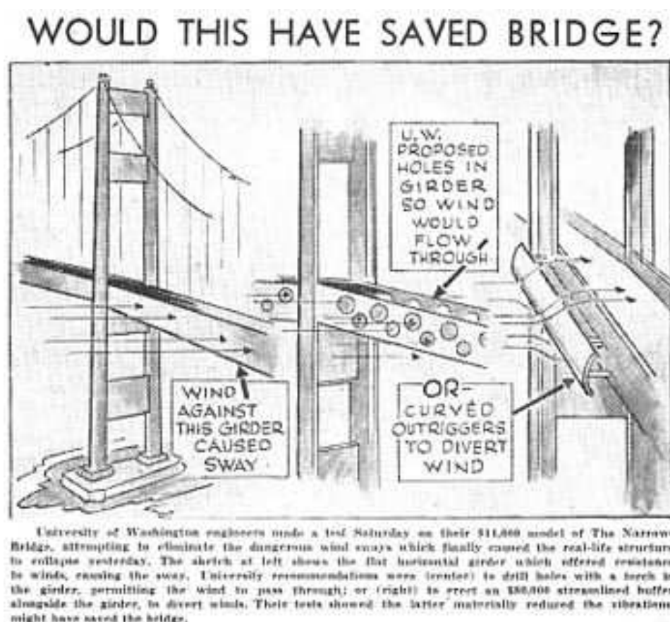
Slika 4. Moguća rješenja za redukciju aerodinamičnih sila na most [4]
