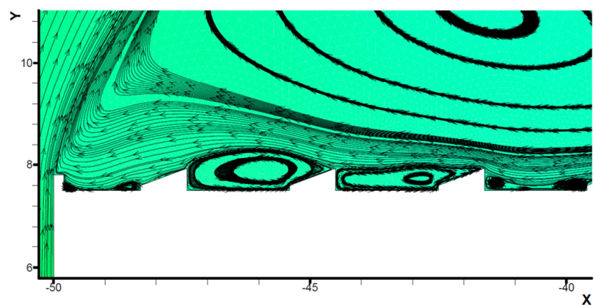
Slika 69. Opstrujavanje oko 1., 2. i 3. reda panela u simulaciji E sa suprotnim smjerom strujanja
