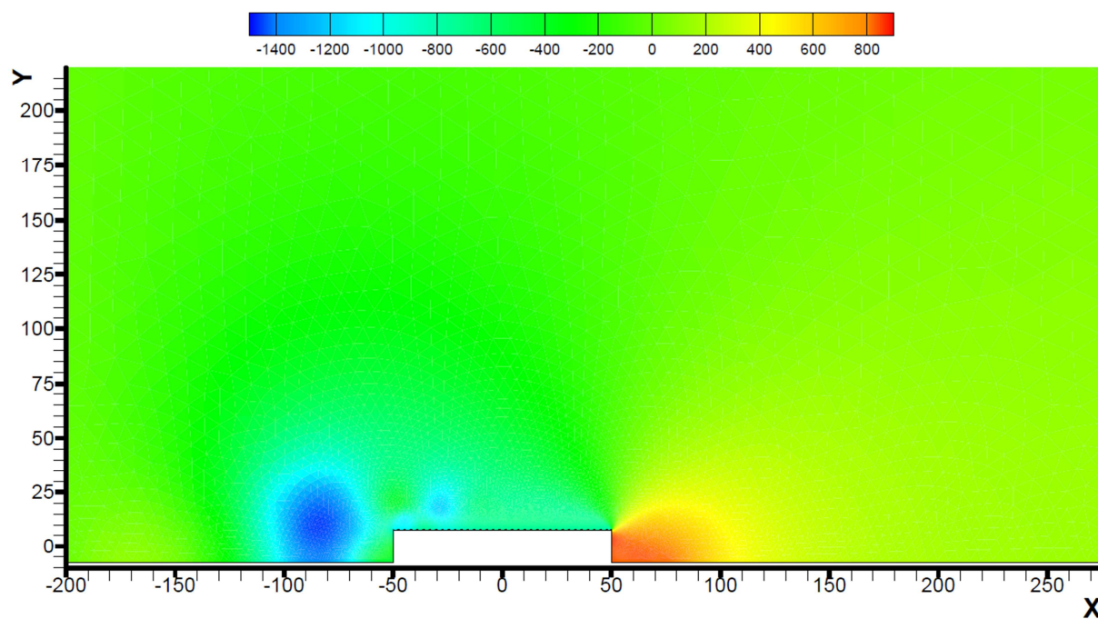
Slika 109. Polje tlaka simulacije I sa suprotnim smjerom strujanja
