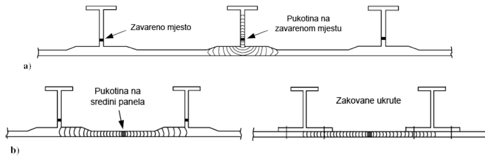
Slika 2-1 Inicijacija pukotine, a) na mjestu zavara, b) na sredini panela [1]
