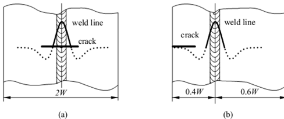
Slika 2-2 Inicijacija pukotine a) na mjestu zavara b) na kraju ploče
