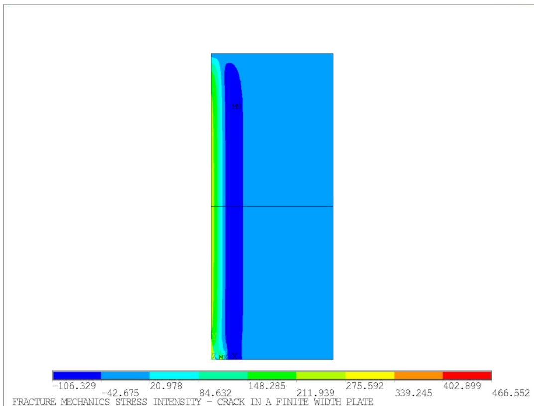
Slika 3-6 Zaostala naprezanja za multilinearu karakteristiku materijala ( a=7.7 mm)
