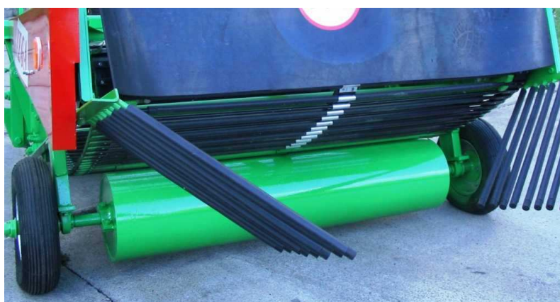
Slika 32 WEGA 1400/1600 gumirane ručice za smanjivanje udarca krumpira u tlo i valjak za zaravnavanje tla
