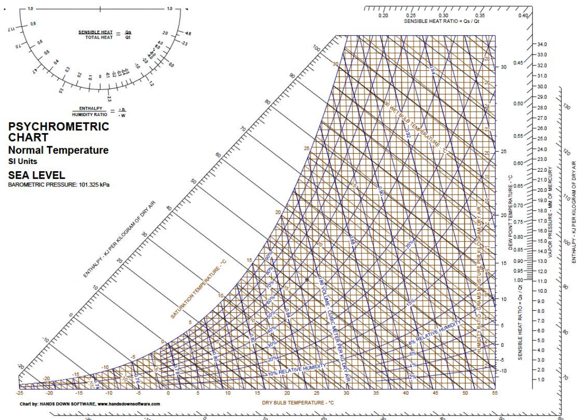
Slika 6 Psihometrijska tablica
