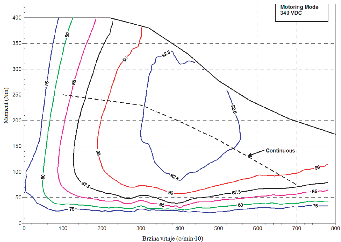
Slika 2.7. Topografski dijagram elektromotora [4]
