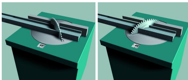
Slika 22. Princip zakretanja [12]
