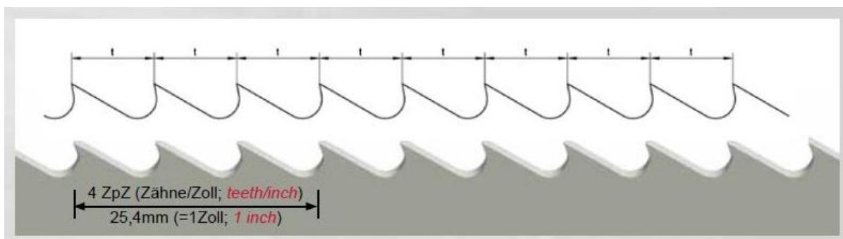
Slika 56. Rezna traka konstantnog koraka [42]
