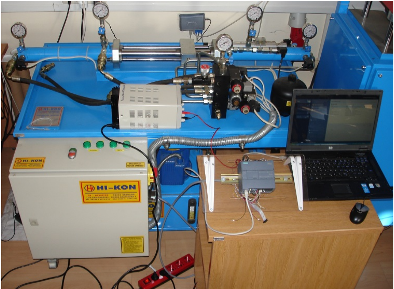
Slika 1: Laboratorijski postav elektrohidrauličkog servosustava
