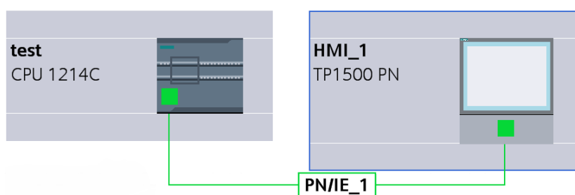
Slika 35: HMI uređaj
