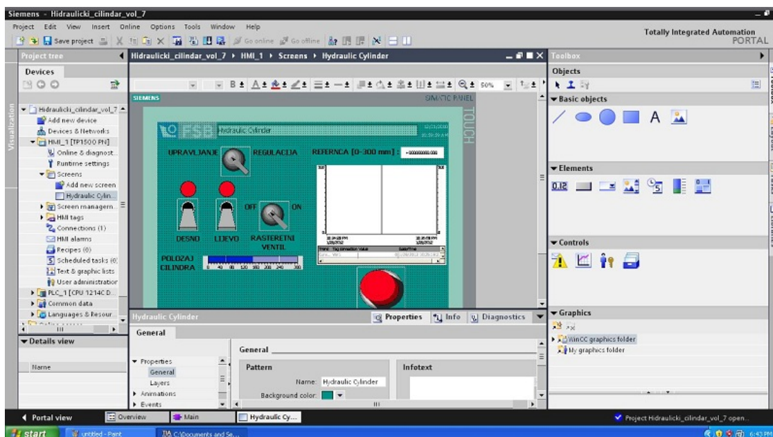
Slika 15: Simatic WinCC
