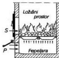
Slika 8. Ravna rešetka
