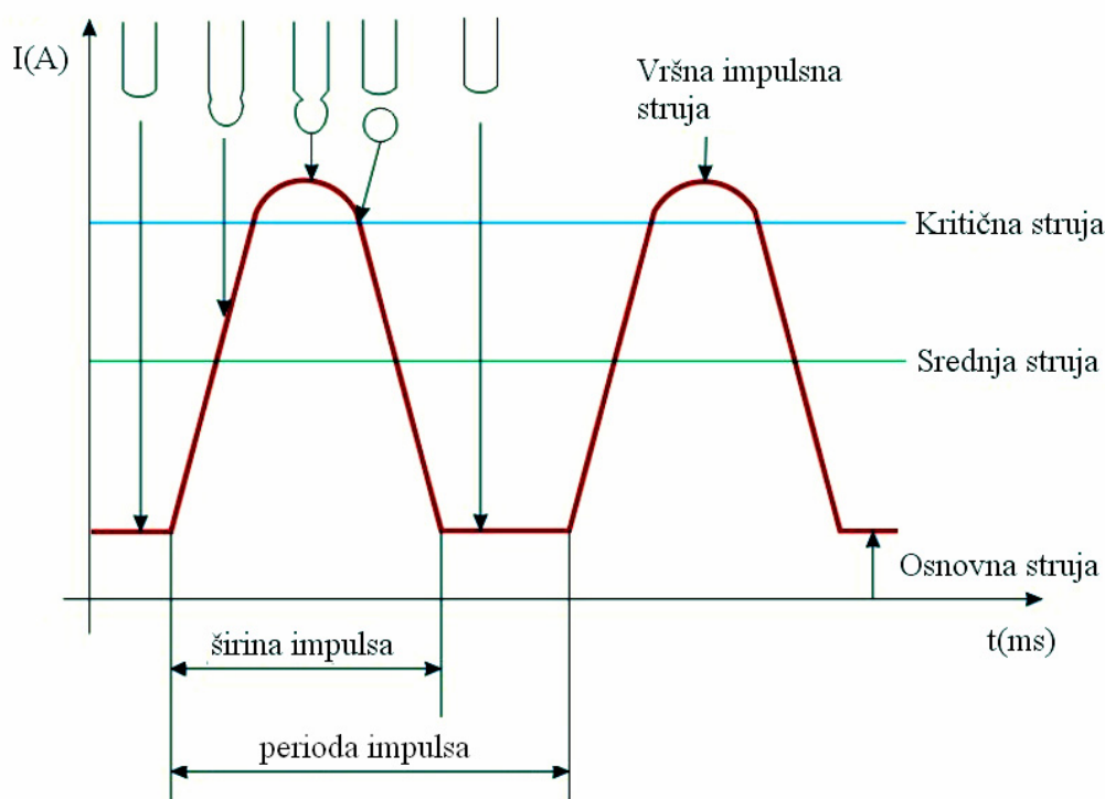
Slika 12. Grafički prikaz impulsnog postupka zavarivanja i otkidanja kapljice [10]
