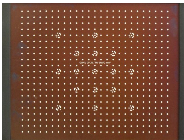
Slika 16. Kalibracijski objekt
