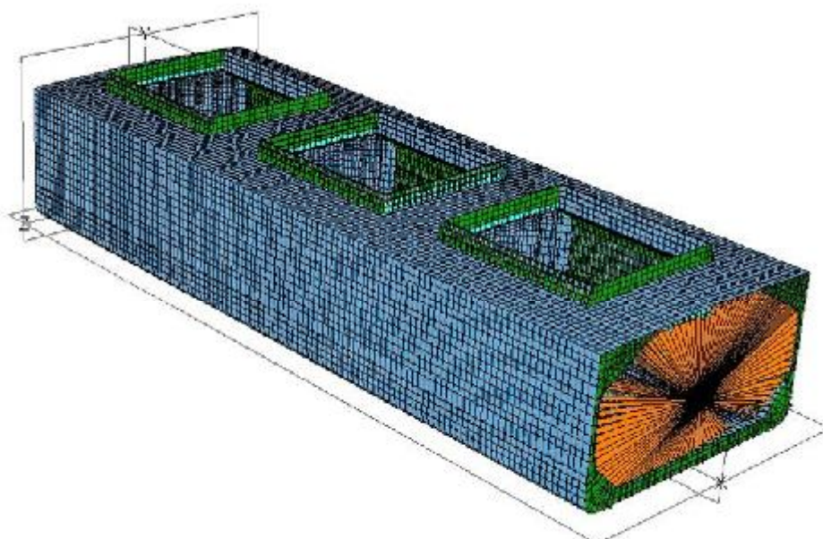
Slika 10. Cijeli MKE model tri skladišta
