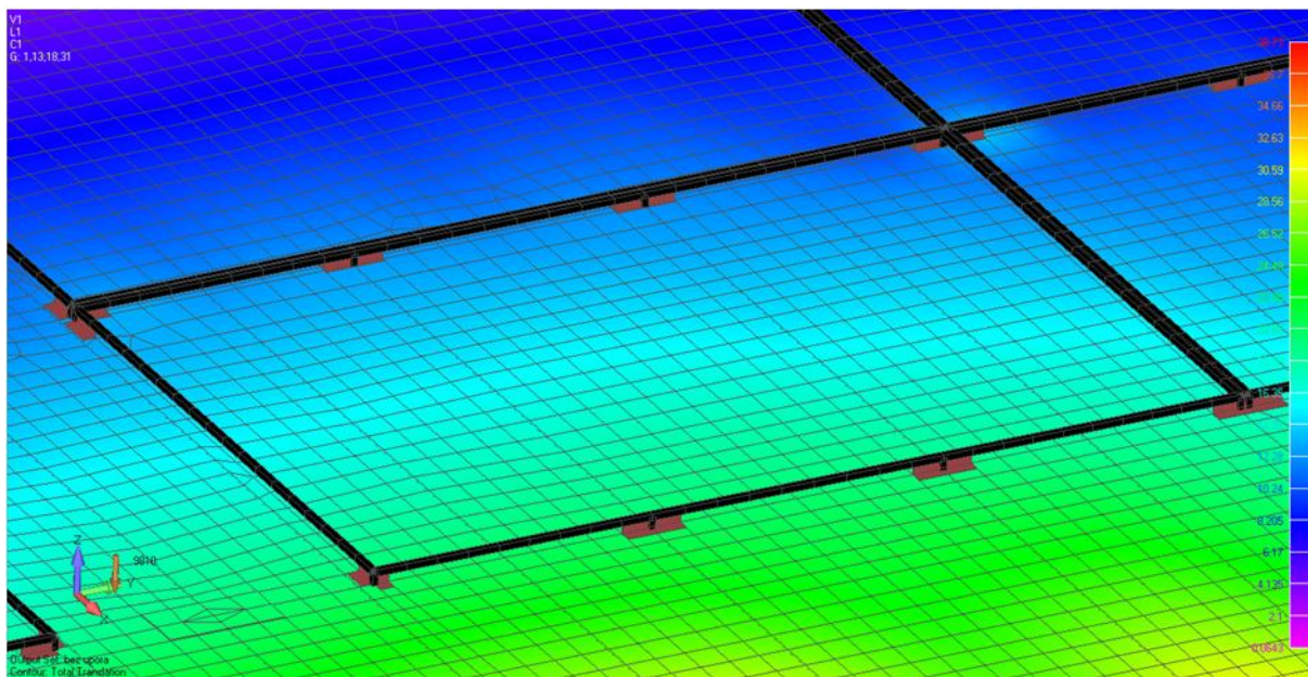
Slika 21. Spoj kabina sa palubom pomoću grednih elemenata
