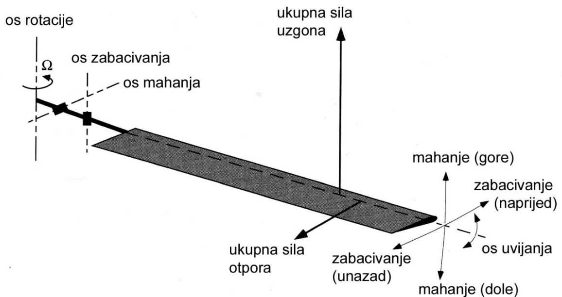
Slika 7 - Prikaz zglobova, sila i kretanja na lopatici rotora
