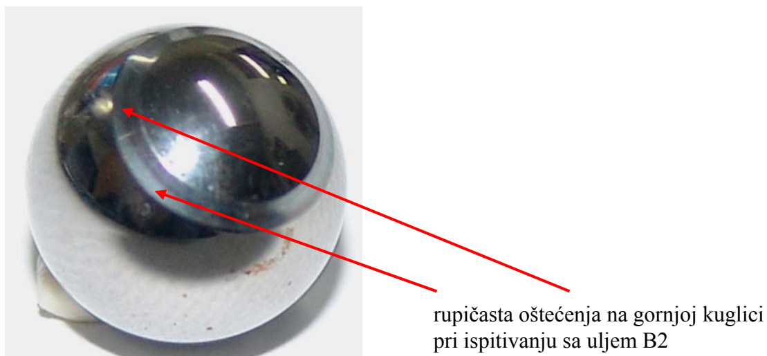
Slika 47. Slika prikazuje rupičasto oštećenje površine kuglice pri mjerenju sa uljem B2
