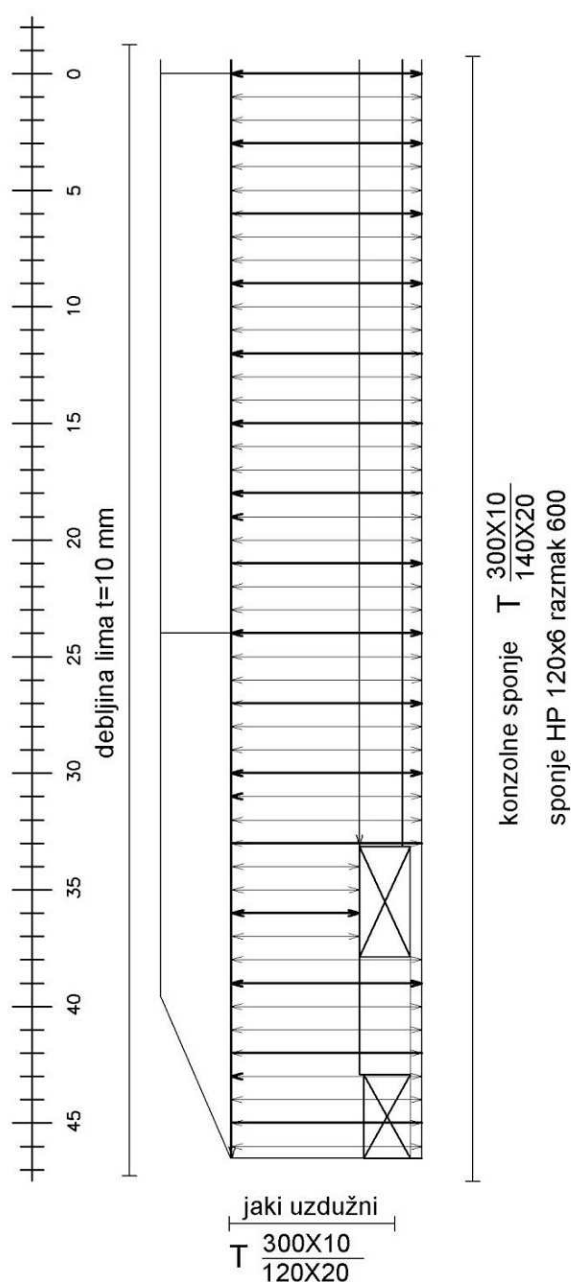
Slika 22: Konstrukcija međupalube
