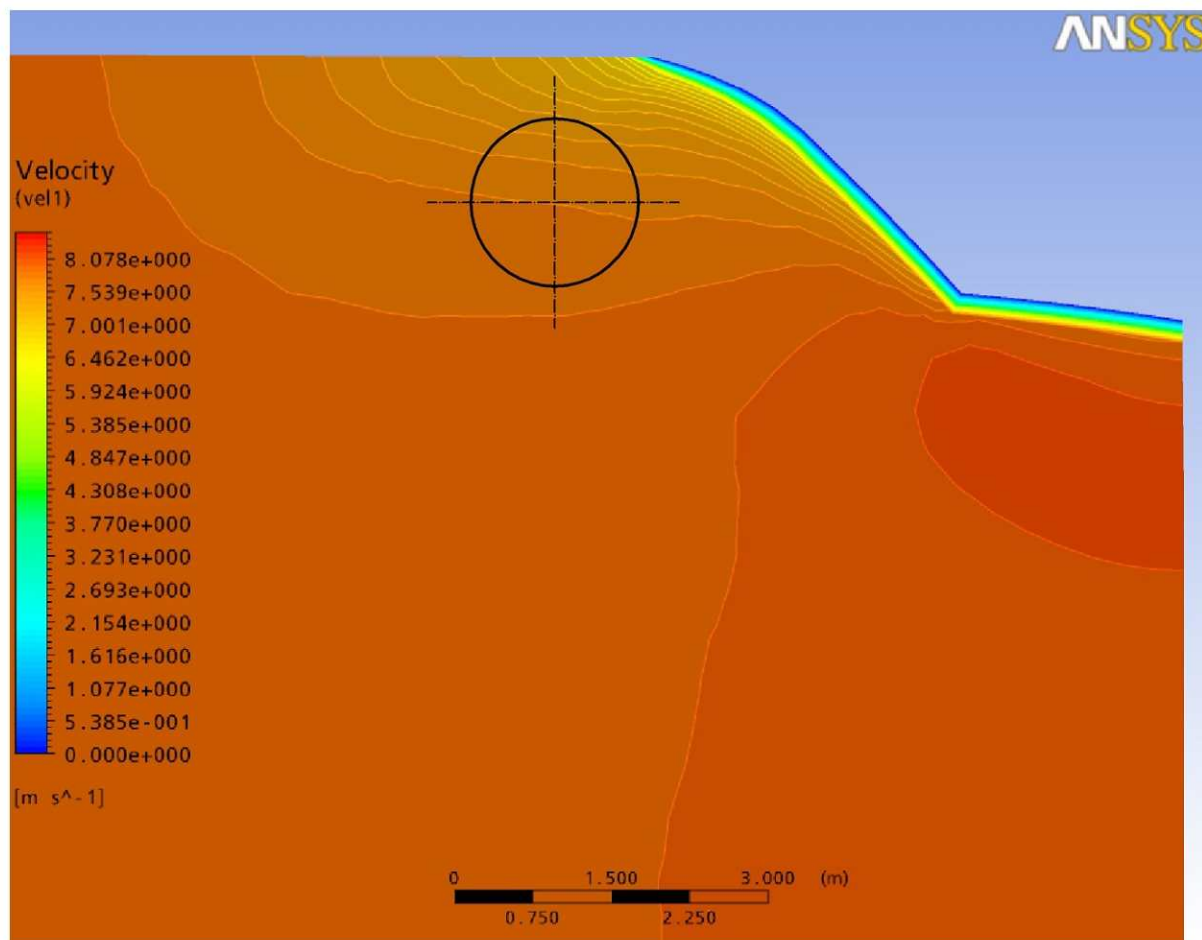
Slika 47: Grafički prikaz brzina u ravni krmelog propelera [S7]
