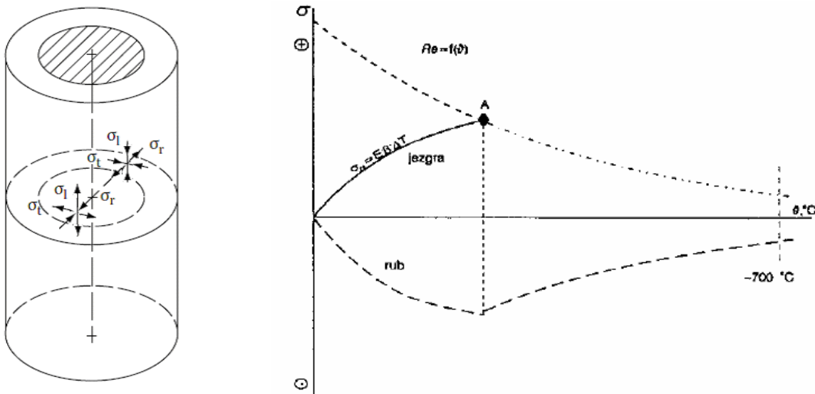
Slika 7. Prikaz nastanka toplinskih naprezanja rubnog sloja i jezgre prilikom ugrijavanja valjka [3],[5]
