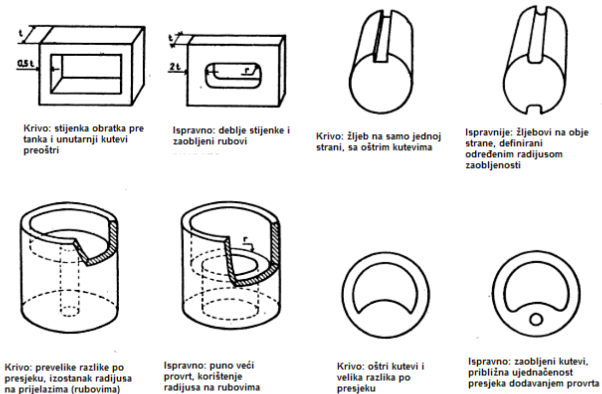
Slika 13. Prikaz nepravilnog i pravilnog oblikovanja obratka za toplinsku obradu [6]
