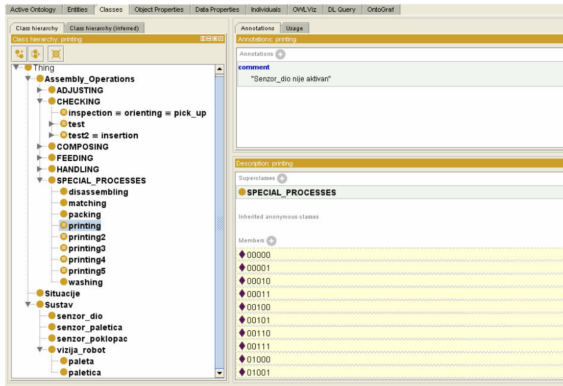
Slika 19. Class hierarchy
