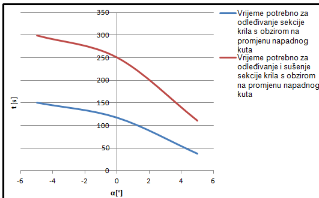
Slika 15. Vrijeme potrebno za odleđivanje i sušenje sekcije krila 1 (bez naštrecavanja vode)
