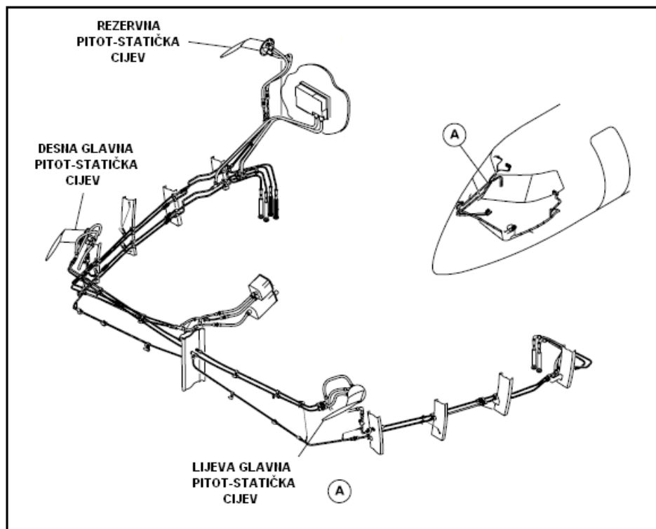
Slika 1-1 Pitot-statički sustav na zrakoplovu Dash Q400 [3]
