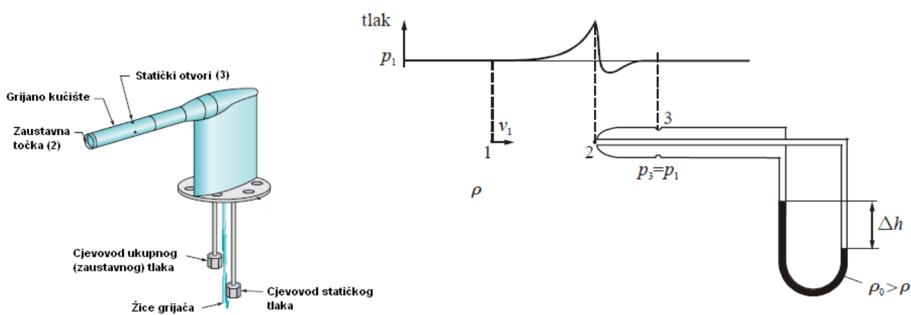
Slika 2-4 Pitot – statička cijev [6], [7]
