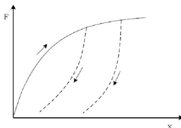
Slika 2.8: Ireverzibilni proces deformiranja asperitnih vlakana
