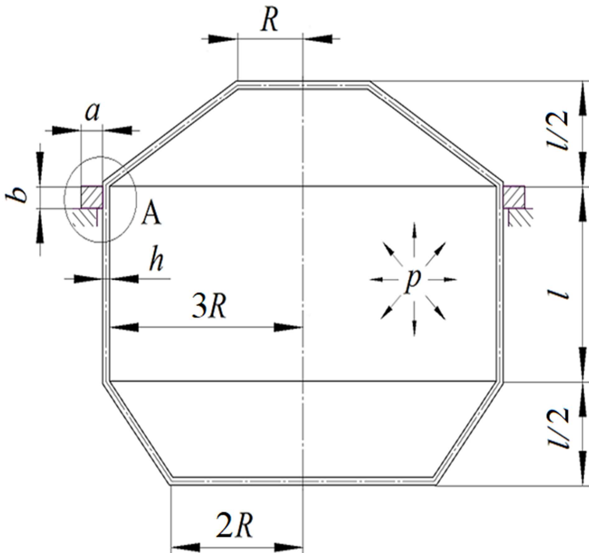
Slika 22. Posuda opterećena unutrašnjim tlakom [9]
