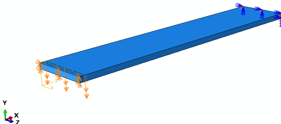
Slika 9. Zadani rubni uvjeti i pomaci (opterećenje)
