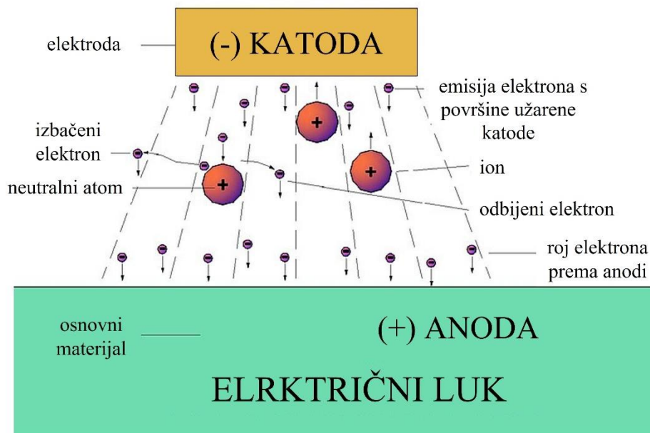
Slika 5. Elektrolučno zavarivanje [32]
