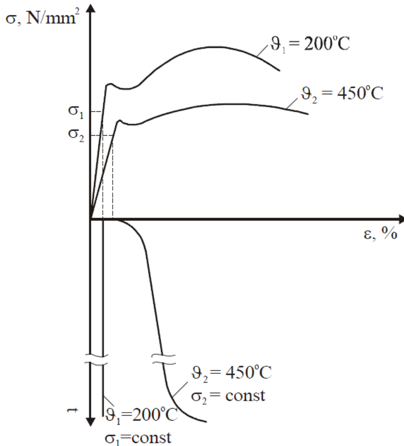
Slika 3 Dijagram naprezanje-produljenje i zakrenuti dijagram puzanja
