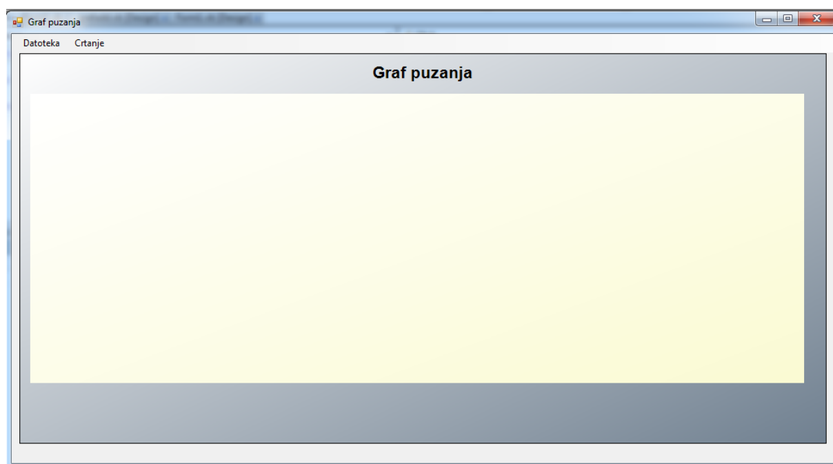
Slika 16 Korisničko sučelje
