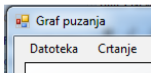
Slika 17 Alatna traka
