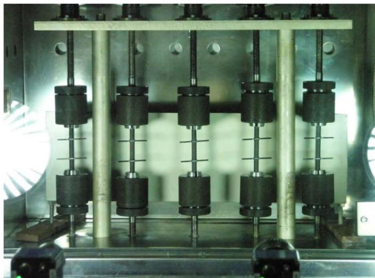
Slika 7 Epruvete pričvršćene u puzalici [3]
