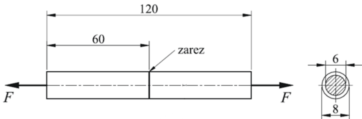
Slika 2 Dimenzije epruvete [3]
