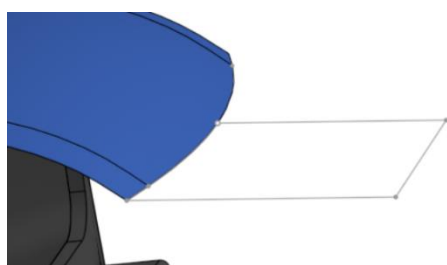
Slika 1057. Rubne krivulje nove površine Nova površina se zrcali oko bočne ravnine ( Right plane ).
