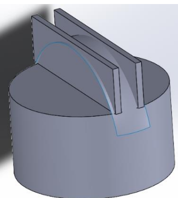
Slika 198. Stvaranje rezne površine
