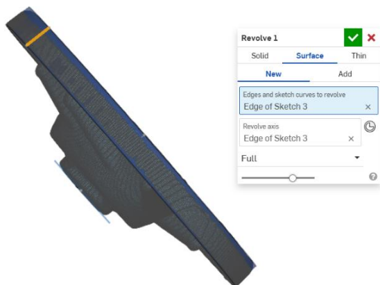
Slika 209. Izrada prve površine alatom Revolve
