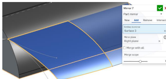
Slika 1092. Zrcaljenje površine
