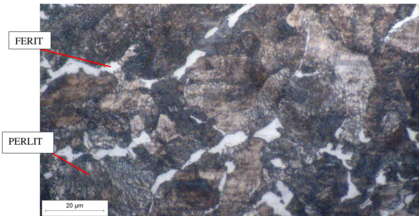
Slika 28. Sredina uzorka, povećanje 1000 x
