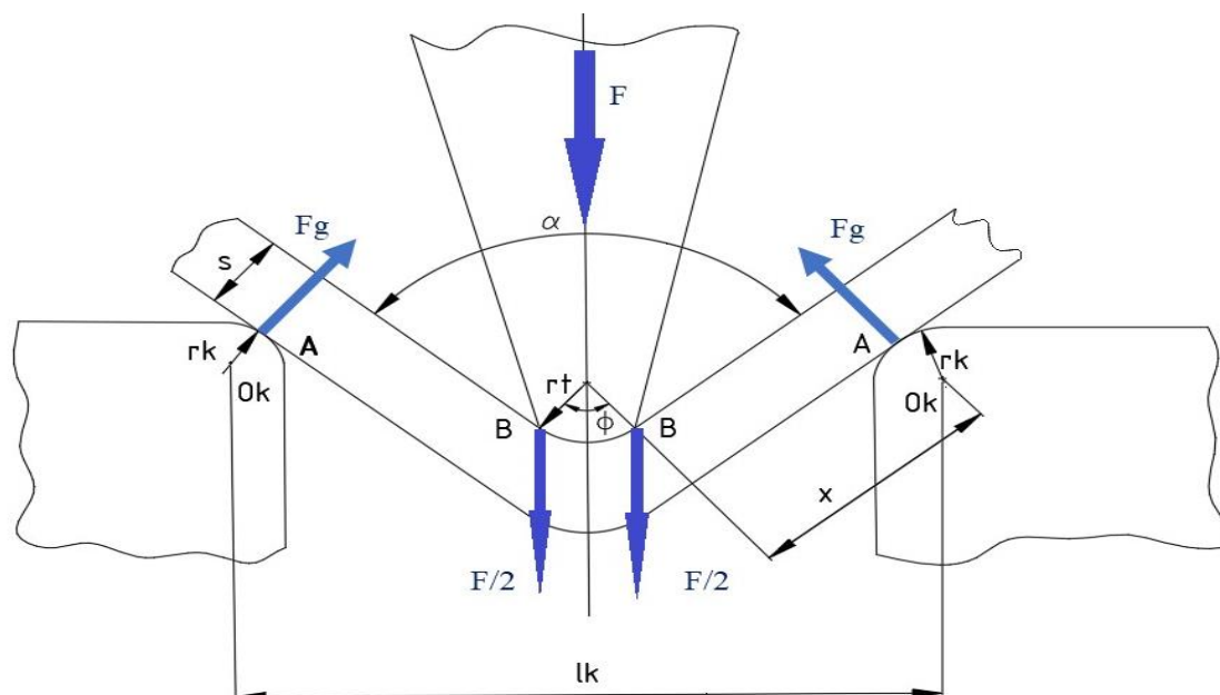
Slika 26. Shema procesa savijanja [5]
