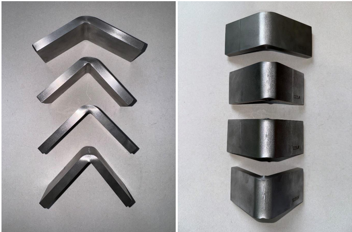
Slika 43. Savijeni komadi - S235JR_10mm
