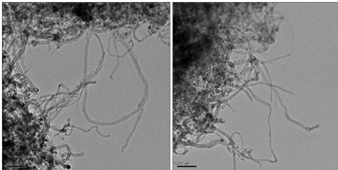
Slika 15 MWCNT snimljene transmisijским elektronskim mikroskopom (TEM) [81].
