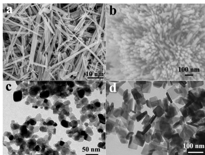
Slika 11 (a) SEM mikrofotografije \text{TiO}_2 nanoštapica; (b) SEM mikrofotografije \text{TiO}_2 nanovrpce; (c) TEM mikrofotografije \text{TiO}_2 Degussa P-25; (d) TEM mikrofotografije Facettailored-a [31].
