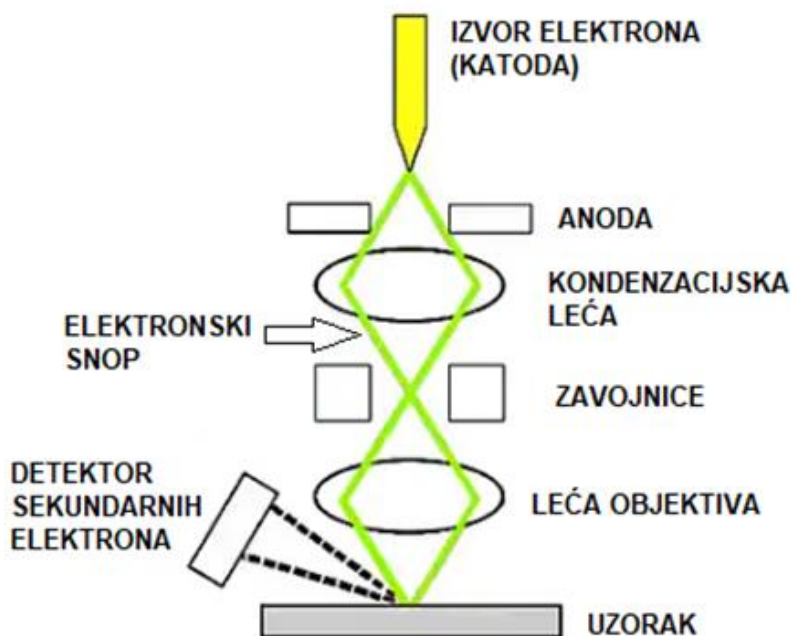
Slika 22 Shematski prikaz principa rada pretražnog elektronskog mikroskopa [110].
