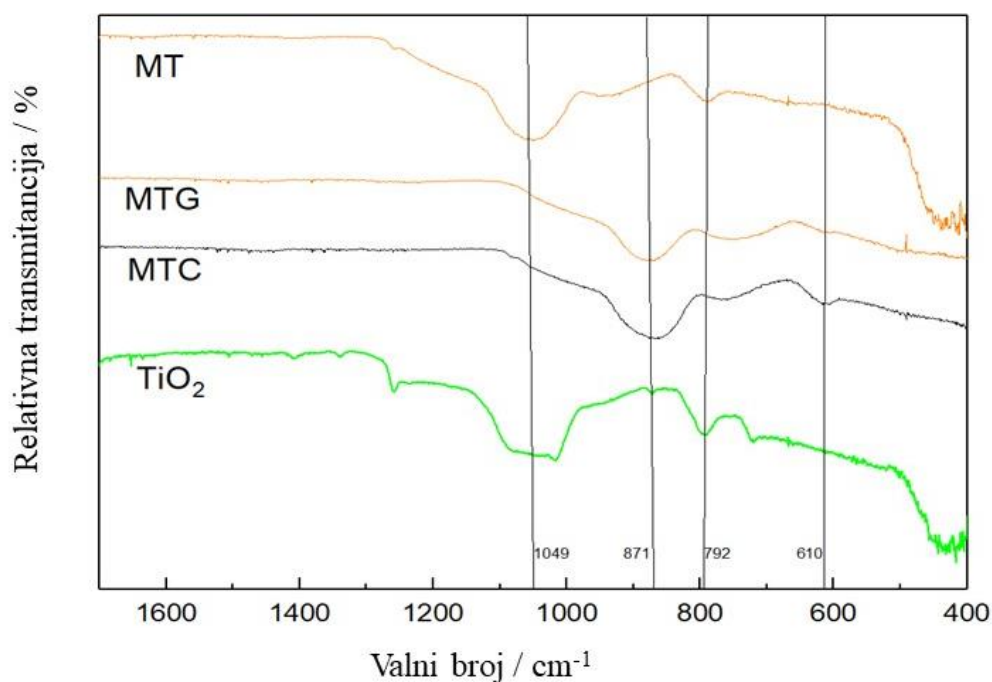
Slika 52 Rezultati FTIR analize imobiliziranih fotokatalizatora na staklenu mrežicu sa karakterističnim vrhovima.
