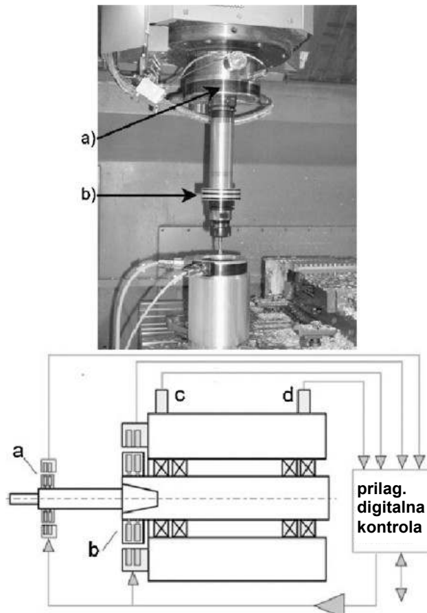
Slika 7.2. Gore: Sustav dvostruke ravnine balansiranja (a: balansirajući prsten na vretenu; b: senzori na statoru); Dolje: Shematski prikaz (a: balansirajući prsten; b: stator sa sensorima za brzinu i položaj; c i d: senzori vibracije) [2]
