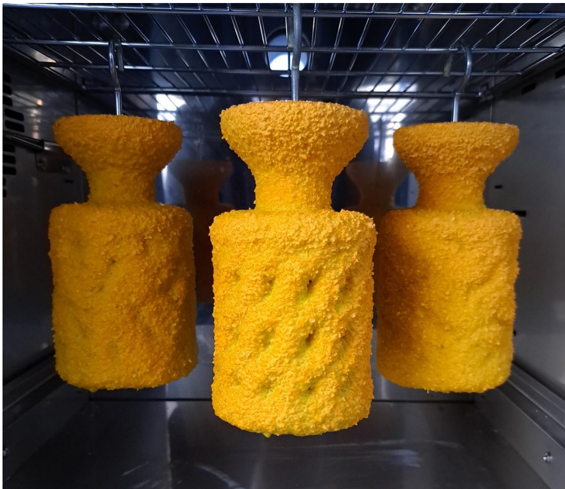
Slika 4.28. Osušene, nežarene keramičke školjke na bazi koloidne silike premazane završnim slojem suspenzije
