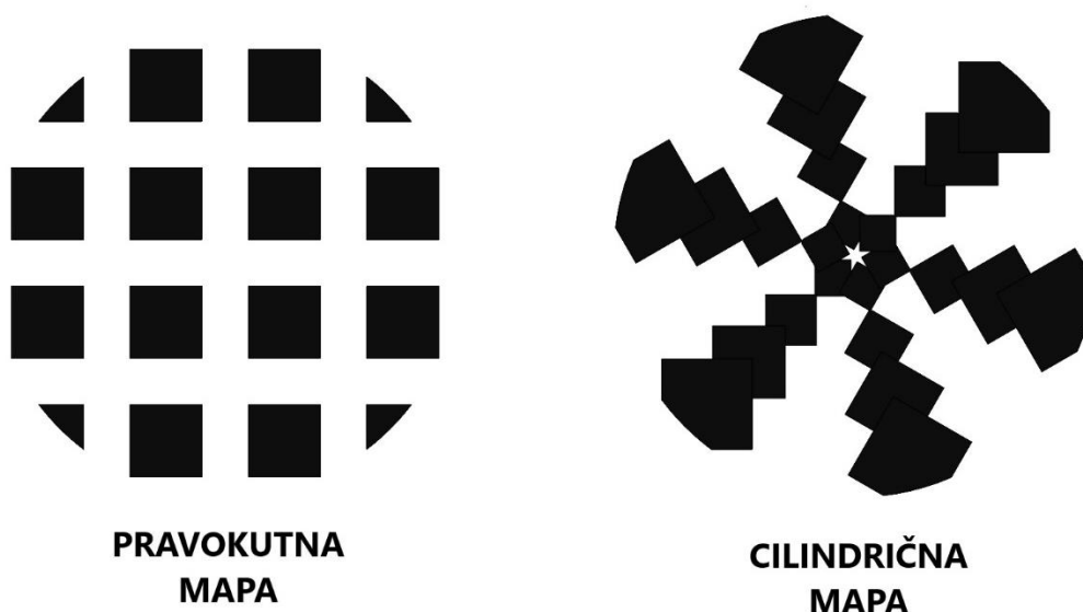
Slika 4.4. Mapiranje ćelija
