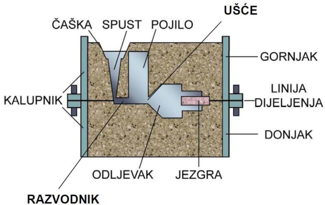
Slika 2.3. Kalup kod pješčanog lijeva [34]
