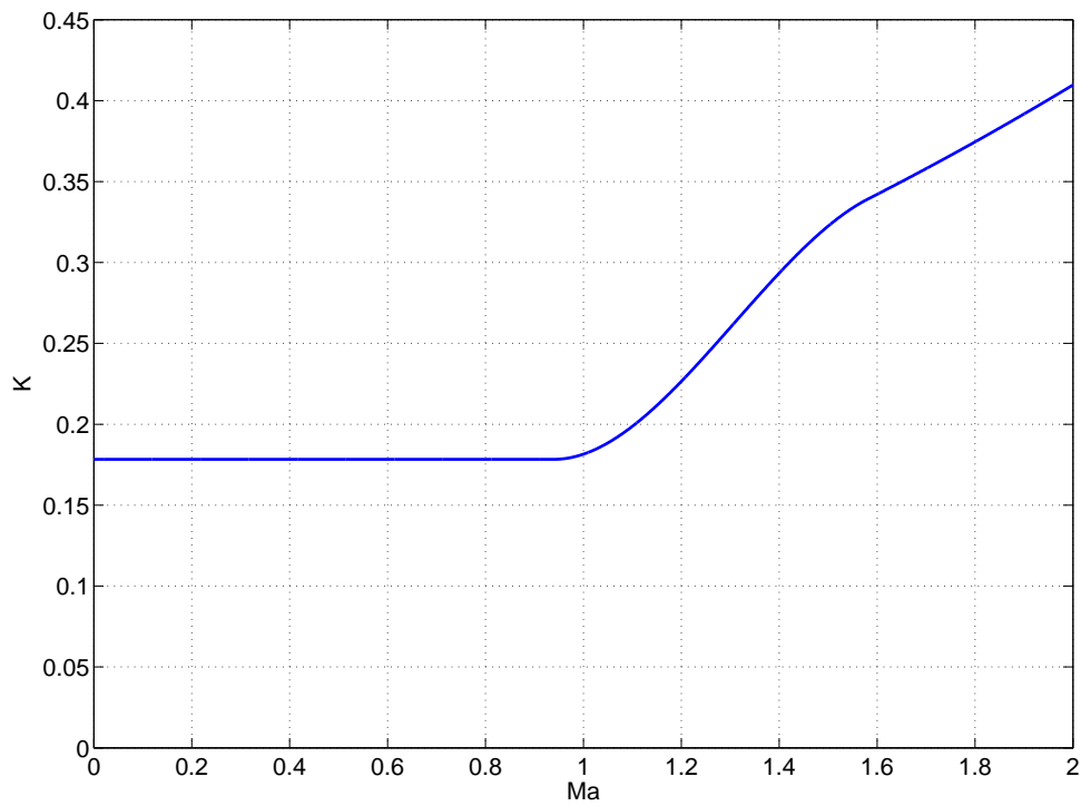
Slika 3.3: Koeficijent induciranoeg otpora - LZ-39
