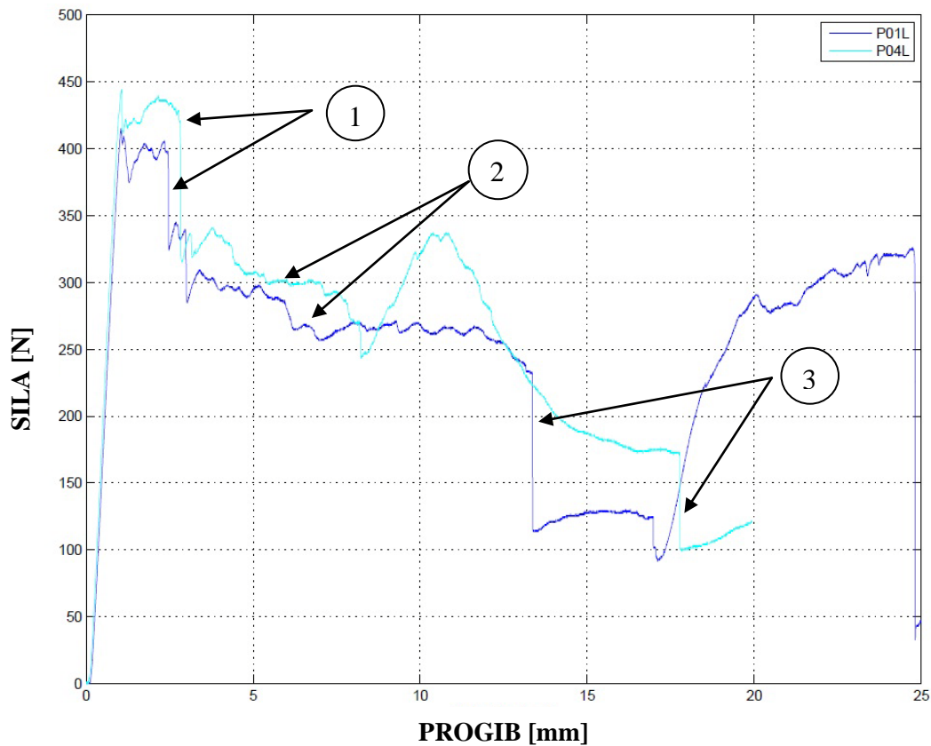
Slika 35. Karakteristične krivulje opterećenje - progib za P-L uzorke
