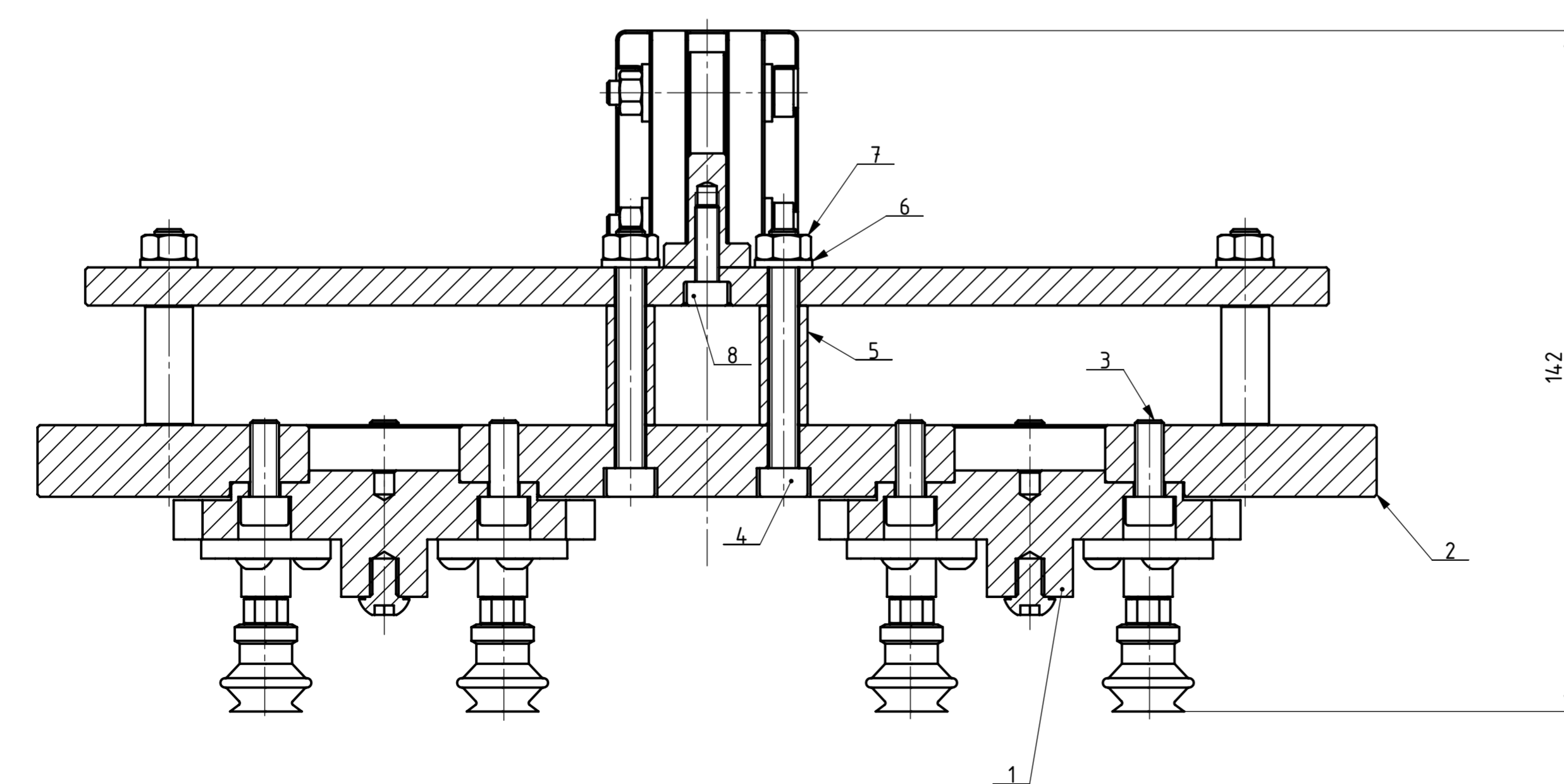
A-A 1:1
