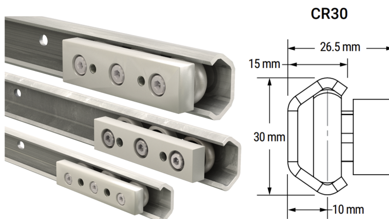
Slika 63. Vodilice CR tvrtke PBC Linear (lijevo) i dimenzije CR30 vodilice (desno) [32]
