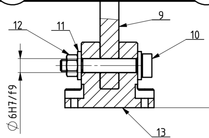
A-A 1:1
