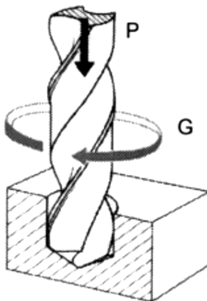
Slika 15. Postupak bušenja s označenim posmičnim (P) i glavnim (G) gibanjem [3]
