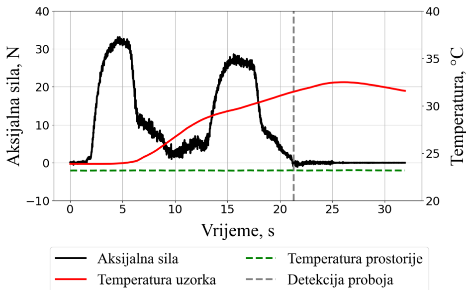
Slika 74. Bušenje Sawbones ploče medicinskim svrdlom ( v_f = 0,5 \text{ mm/s} , d_1 = 3,6 \text{ mm} , \omega = 15^\circ , 2\varphi = 80^\circ )
