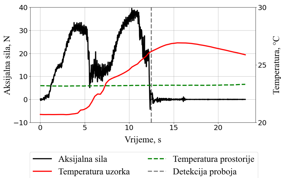
Slika 56. Bušenje teleće lopatične kosti ( v_f = 0,5 mm/s, d_1 = 4,5 mm, \omega = 30^\circ , 2\varphi = 118^\circ )
