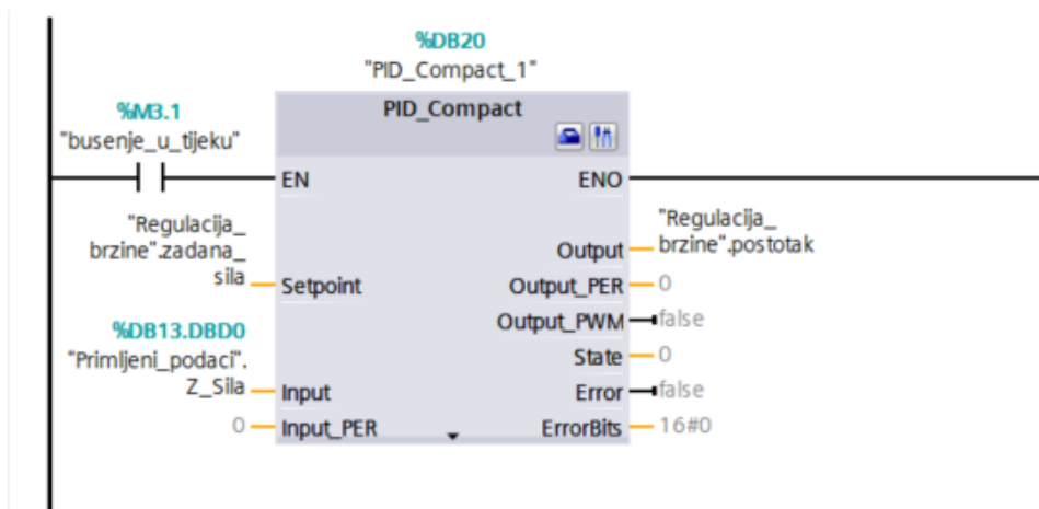
Slika 76. Instrukcija PID_Compact
