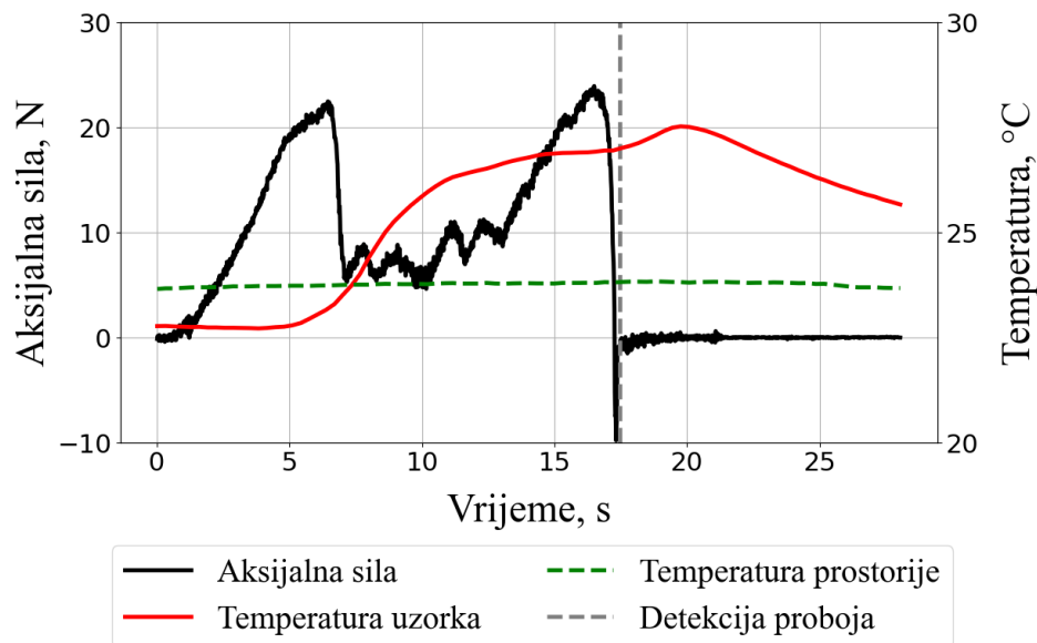
Slika 54. Bušenje teleće lopatične kosti industrijskim svrdlom ( v_f = 0,5 \text{ mm/s} , d_1 = 3 \text{ mm} , \omega = 30^\circ , 2\varphi = 130^\circ )
