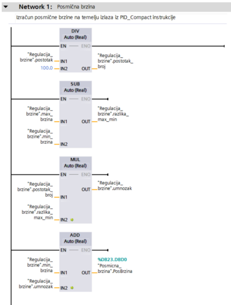
Slika 77. Funkcija za izračun vrijednosti posmične brzine
