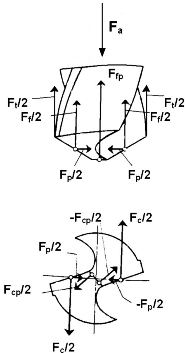
Slika 19. Sile rezanja [7], [8], [9]
