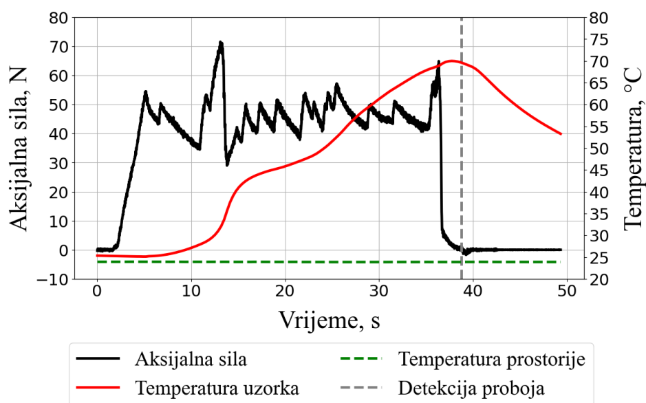
Slika 57. Bušenje teleće lopatične kosti medicinskim svrdlom ( v_f = 0,5 \text{ mm/s} , d_1 = 2,5 \text{ mm} , \omega = 15^\circ , 2\varphi = 80^\circ )
