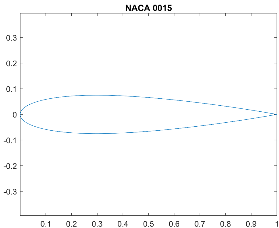
Slika 14. NACA 0015
