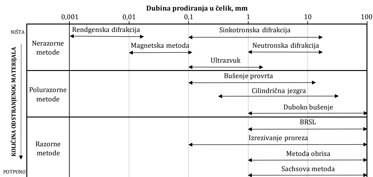
Slika 21. Podjela metoda mjerenja zaostalnih naprežanja [30]
