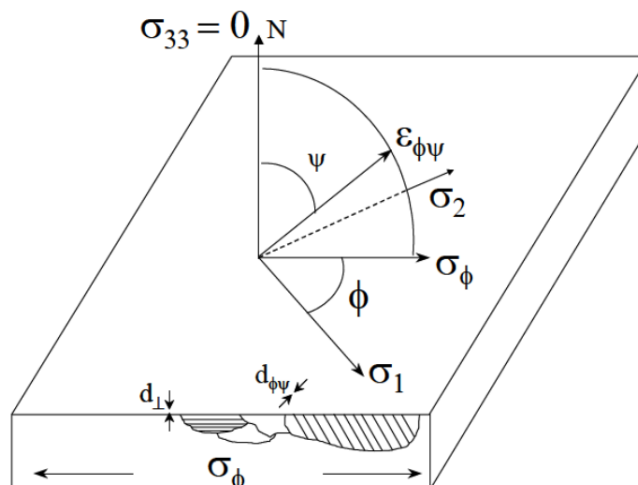
Slika 23. Shema uzorka u ravninskom stanju napreznja s prikazom različitih orijentacija kristalnih ravnina [32]
