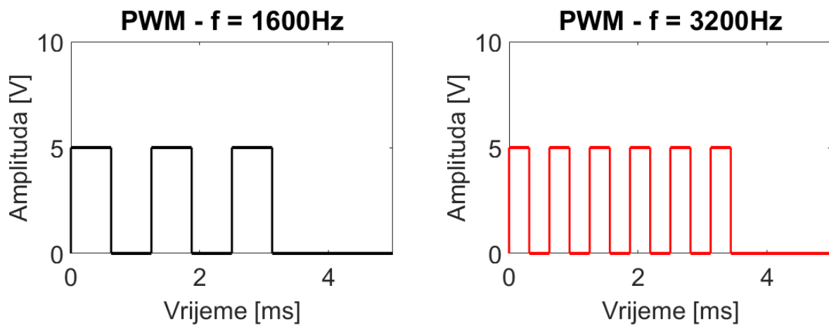
Slika 47 Vizualizacija dva PWM signala
