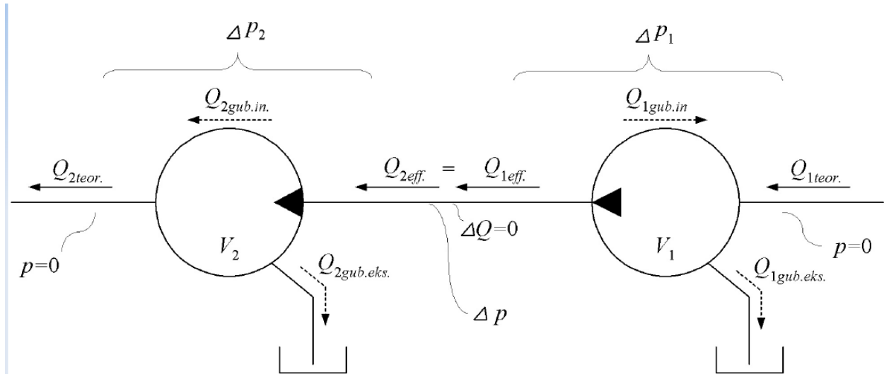
Slika 3.7. Hidromehanički gubici [5]
