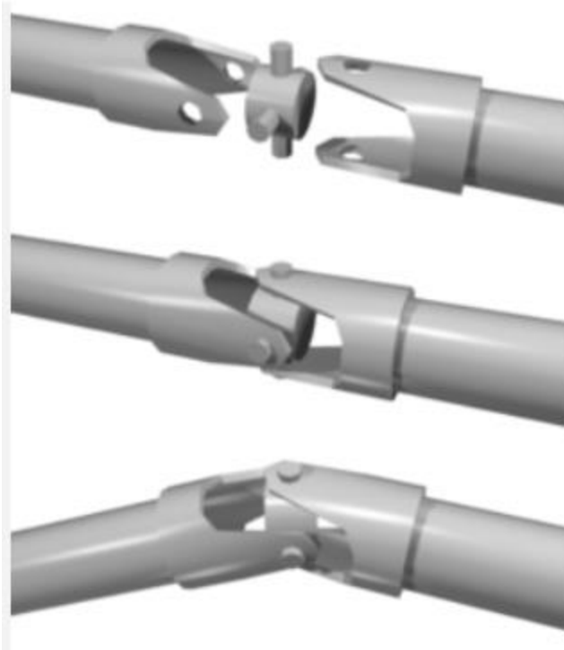
Slika 1.1. Kardansko vratilo [2]
