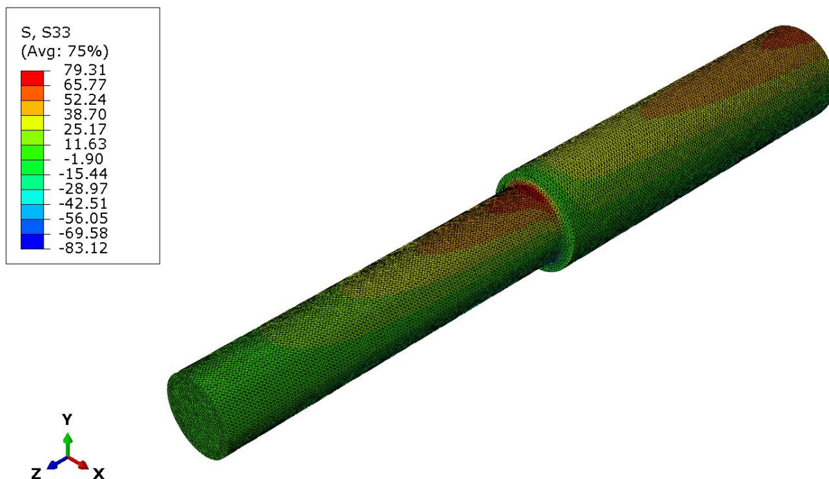
Slika 37. Prikaz rezultata numeričke analize modela opterećenog na uvijanje (651968 elemenata)
