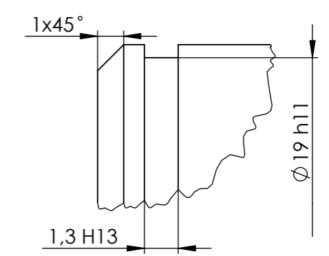
Detalj D M 5:1
