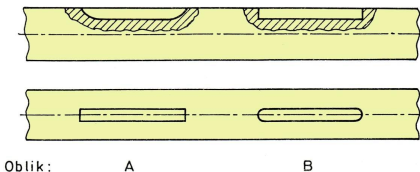
Slika 27. Faktor zareznog djelovanja kod savijanja vratila s utorom za pero [5]
