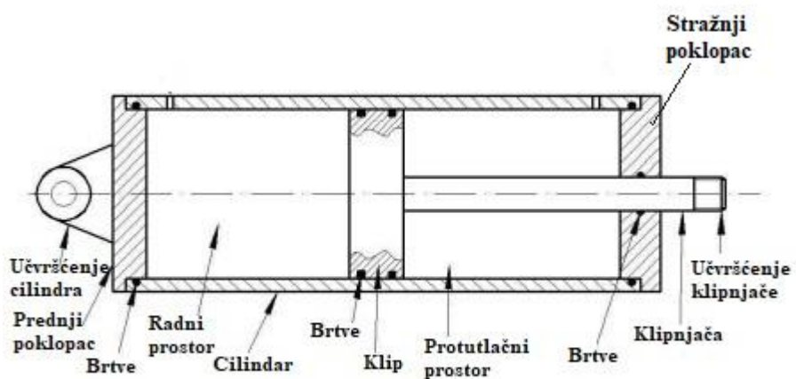
Slika 12. Dijelovi hidrauličnog cilindra [27]
