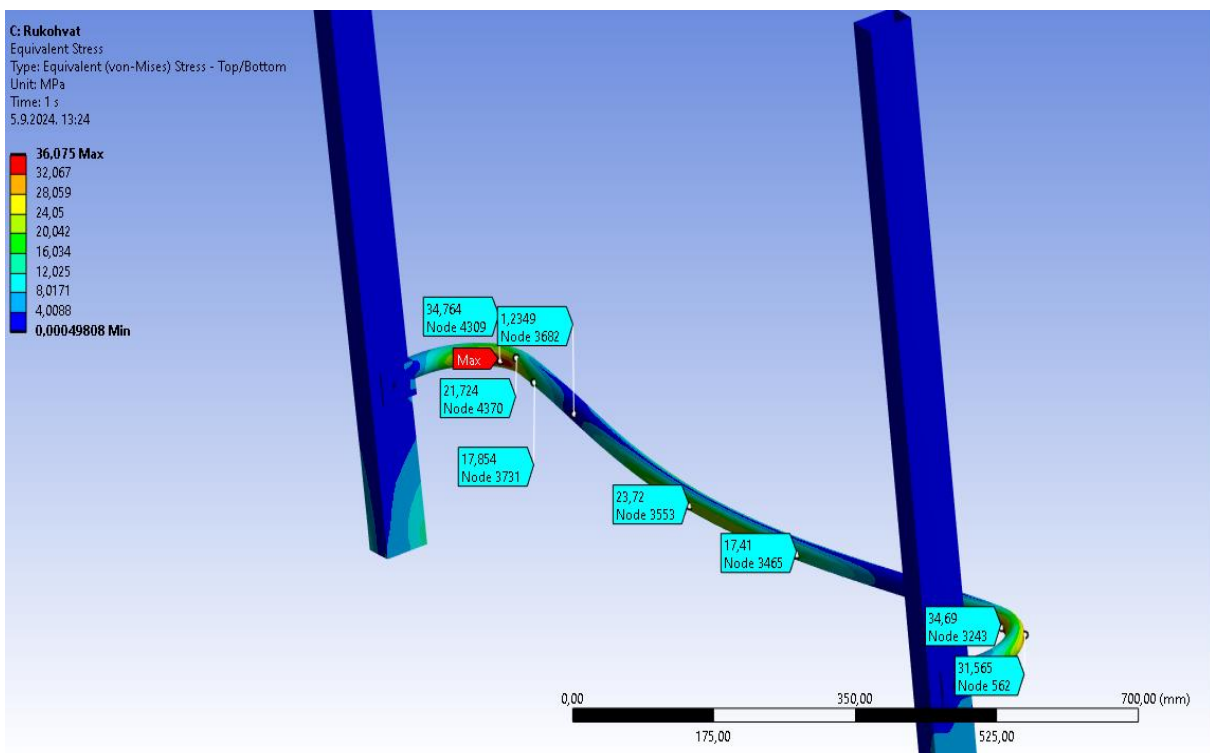
Slika 60. Rezultat naprezanja rukohvata
