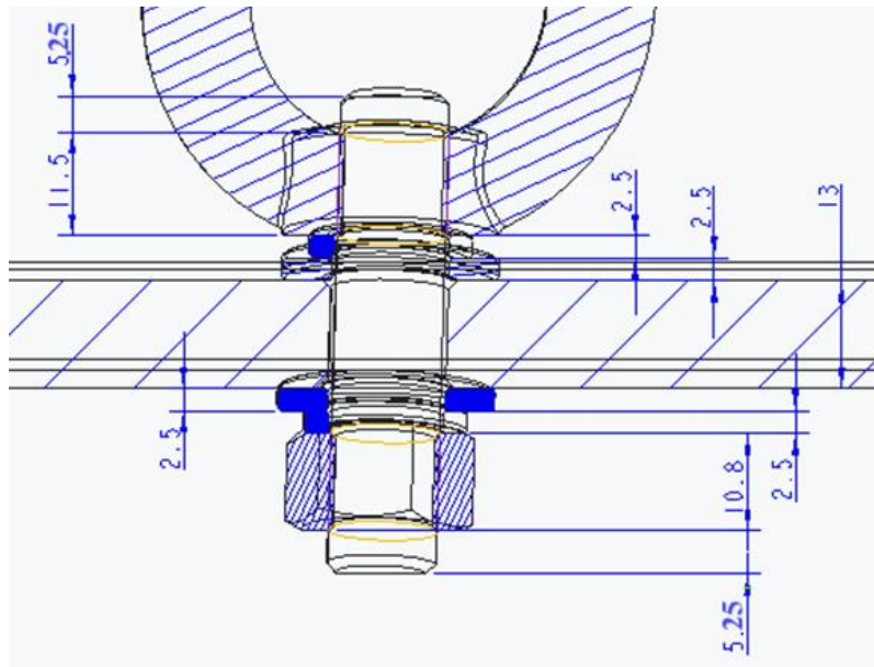
Slika 49. Dimenzije komponenata na vijku
