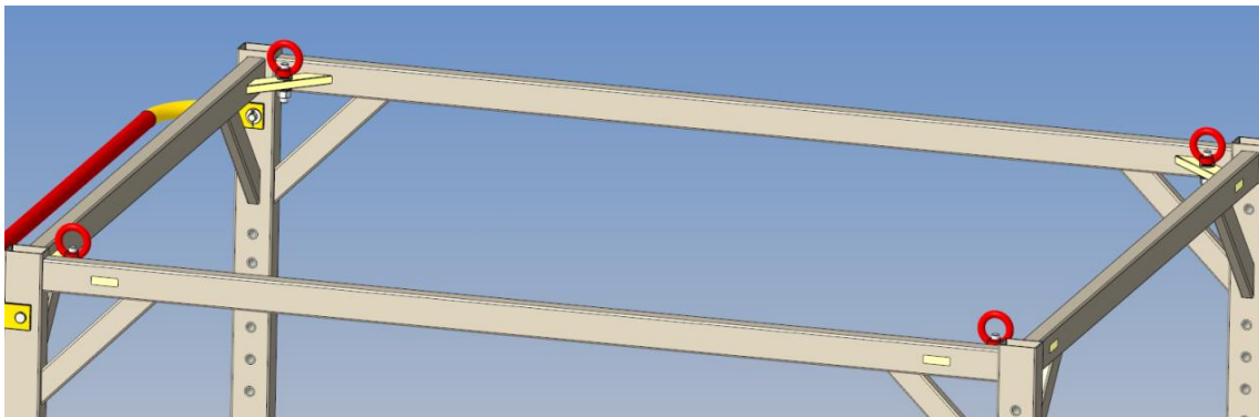
Slika 50. Ušice i ukrute
