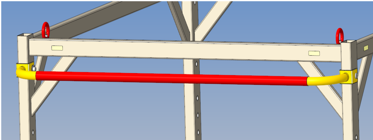
Slika 38. Konstrukcijsko rješenje rukohvata
