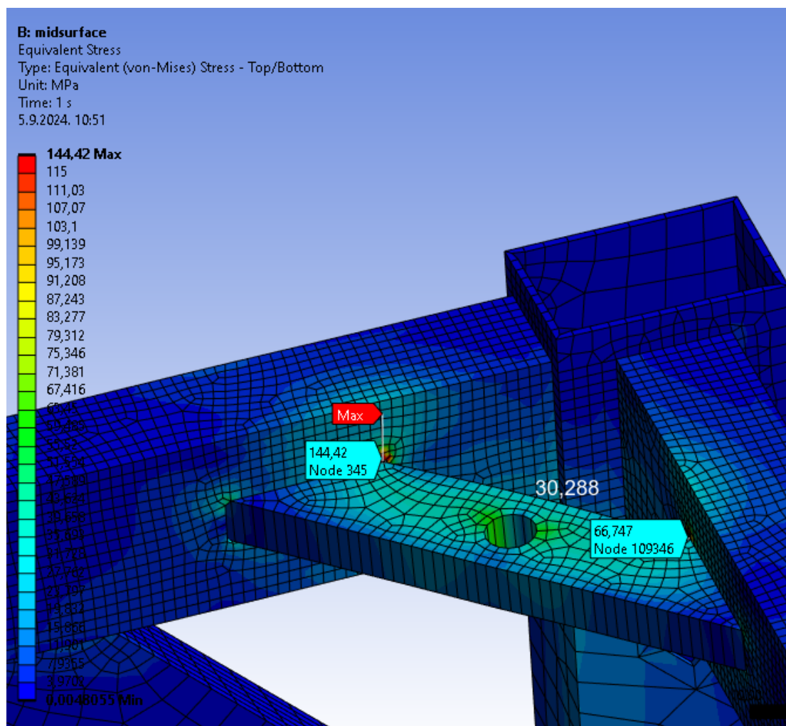
Slika 58. Kritična zona s gušćom mrežom konačnih elemenata
