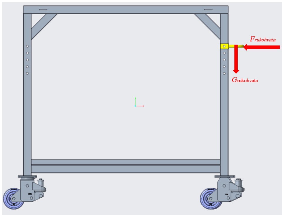
Slika 34. Opterećenje svornjaka
