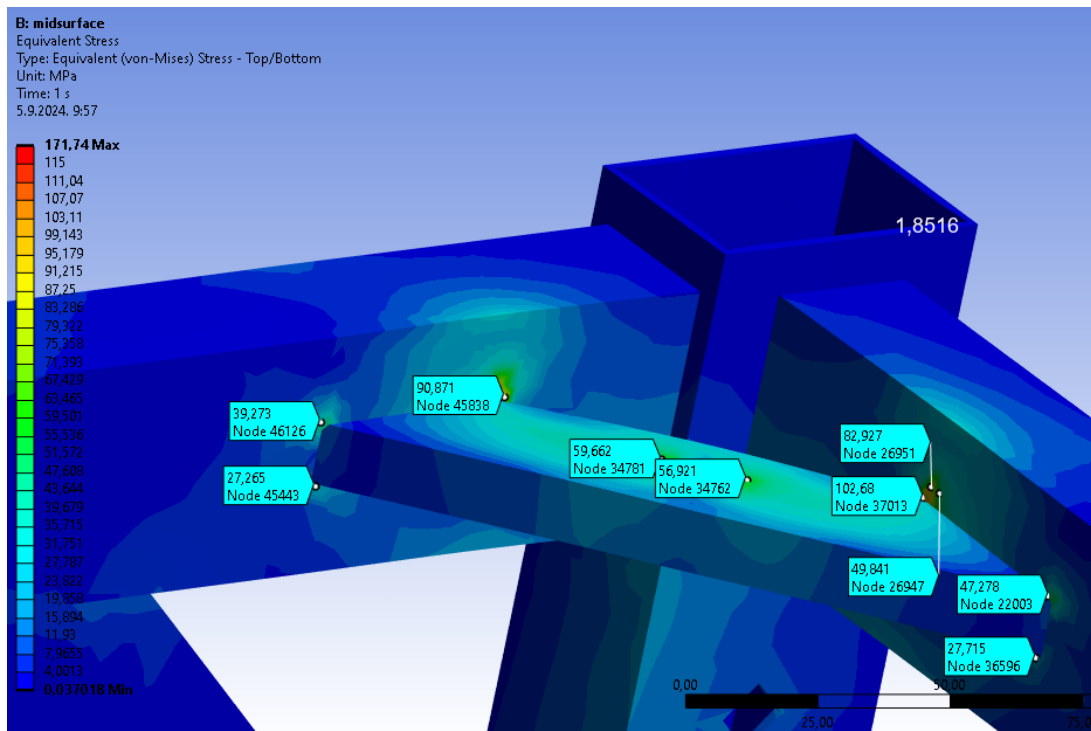
Slika 56. Naprezanje ukrute za prihvat očnog vijka
