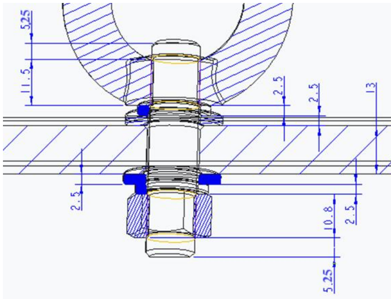
Slika 49. Dimenzije komponenta na vijku
