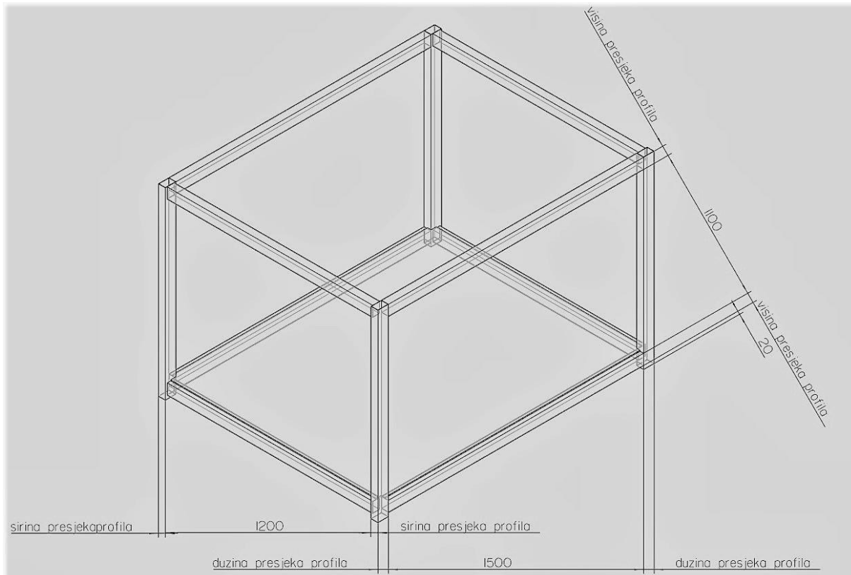
Slika 10. Mreža kaveza
