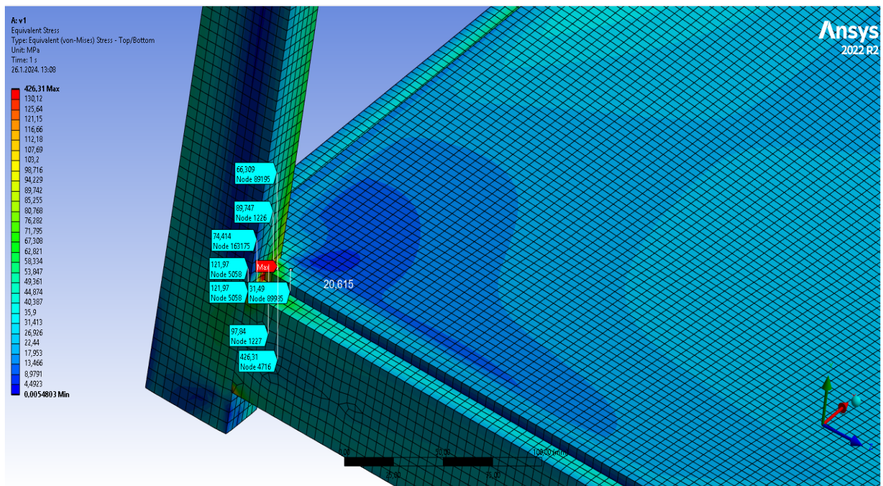
Slika 16. Napreznje u oko mjesta koncentracije napreznja
