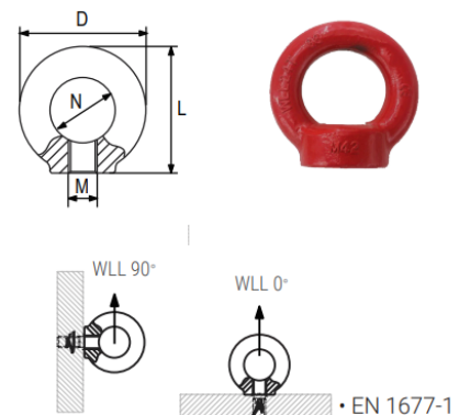
Slika 45. Tablica karakteristika odabrane ušice [25]
