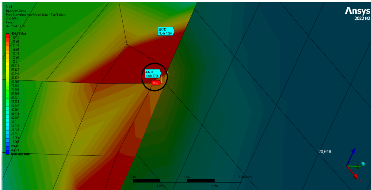
Slika 15. Mjesto koncentracije napreznja
