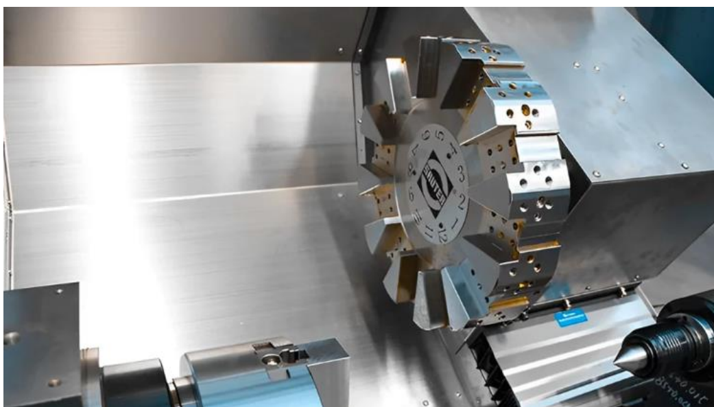
Slika 24. Revolverska glava bez postavljenih alata [28]
