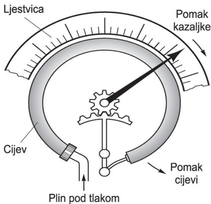
Slika 4. Bourdonova cijev
