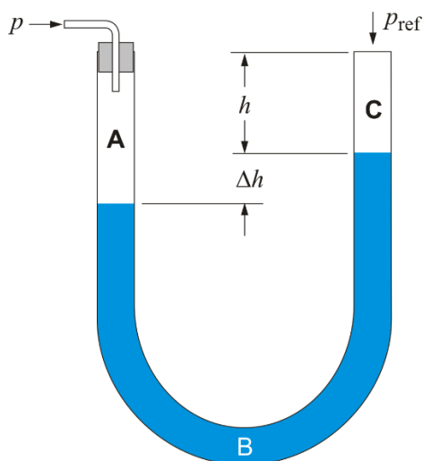
Slika 3. U-manometar
